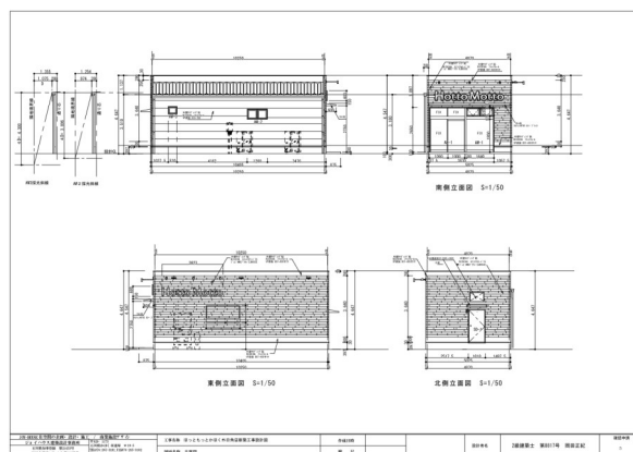
設計図
